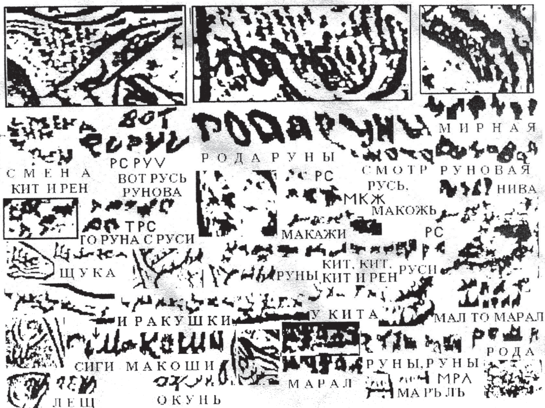
Чтение надписей
